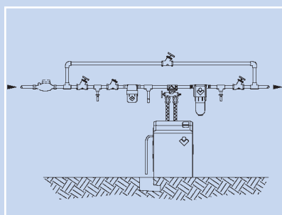
Ejemplo de instalación para aguas potables
